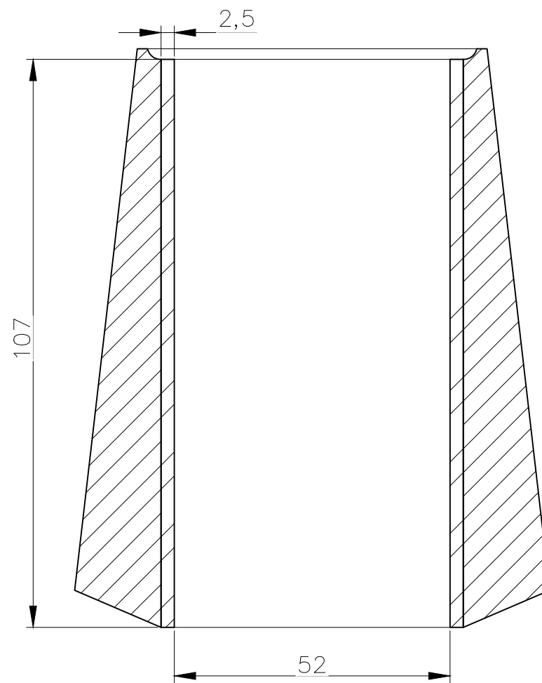
SECTION A-A
